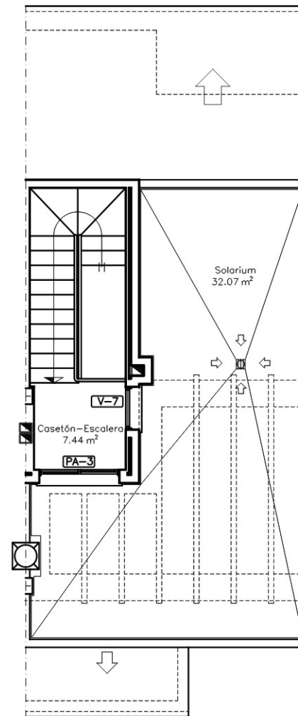
PLANTA SOLARIUM MOBILIARIO Y SUPERFICIES
