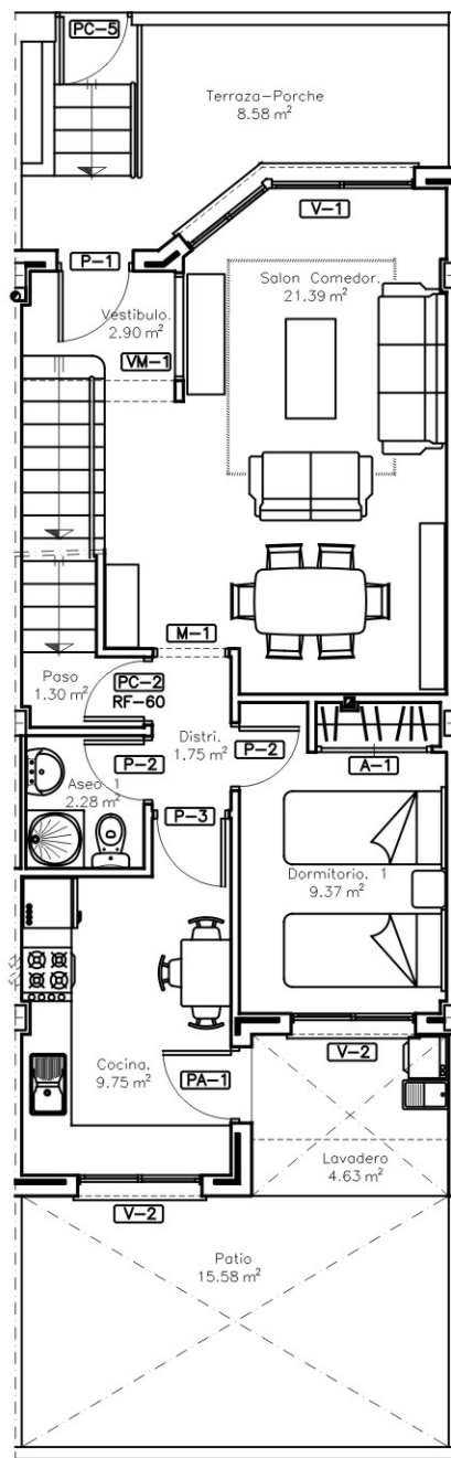
PLANTA BAJA MOBILIARIO Y SUPERFICIES
