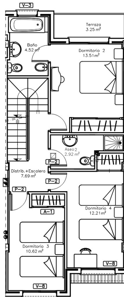
PLANTA PRIMERA MOBILIARIO Y SUPERFICIES
