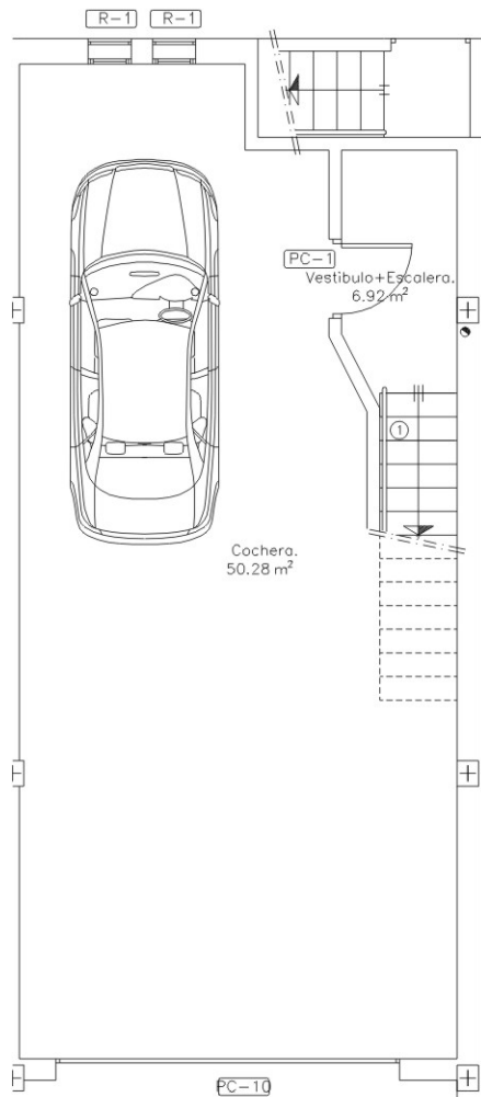
PLANTA SEMISOTANO MOBILIARIO Y SUPERFICIES
