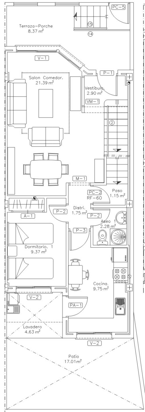
PLANTA BAJA MOBILIARIO Y SUPERFICIES
