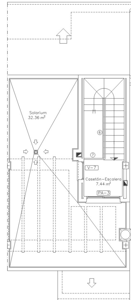
PLANTA SOLARIUM MOBILIARIO Y SUPERFICIES
